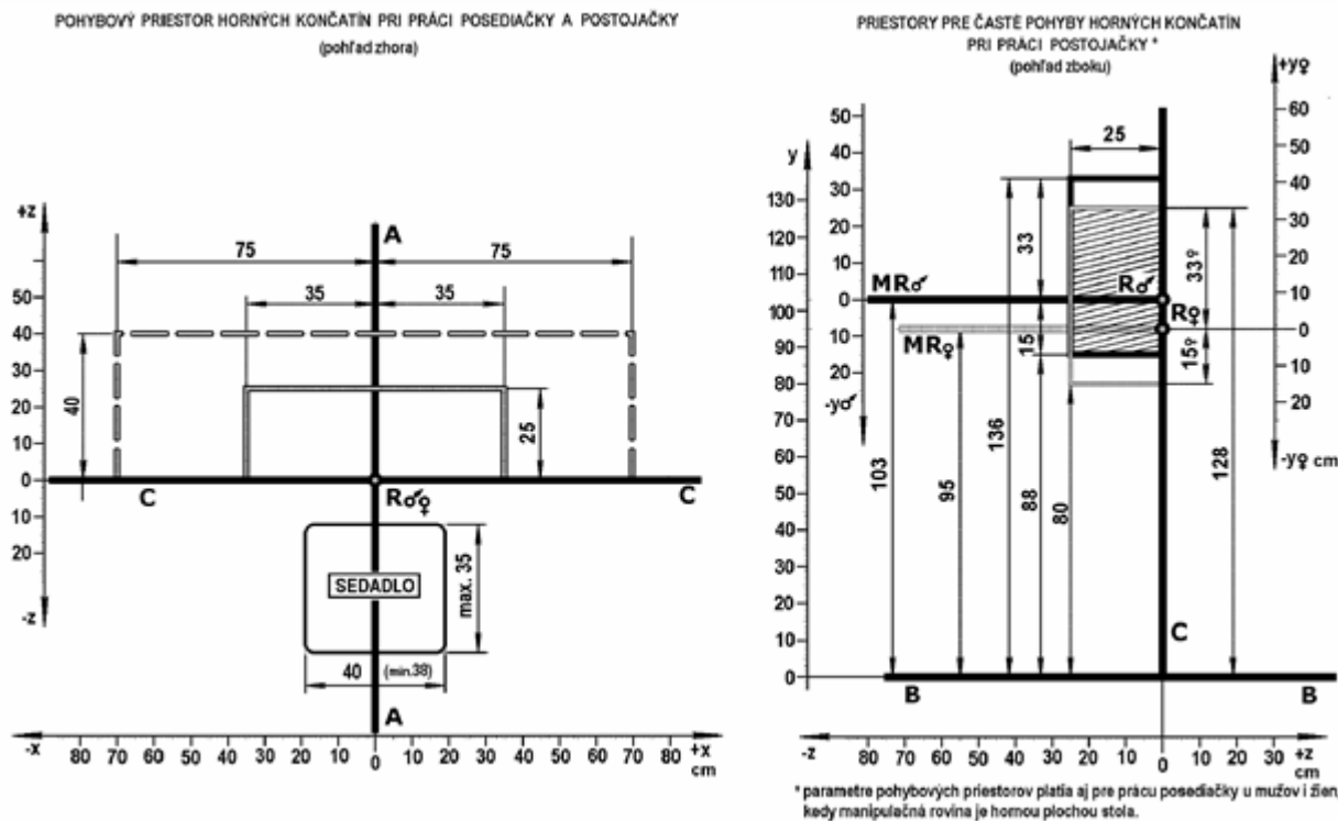
Obrázok č. 3 Priestor pre pohyby horných končatín pri práci Vysvetlivky:
